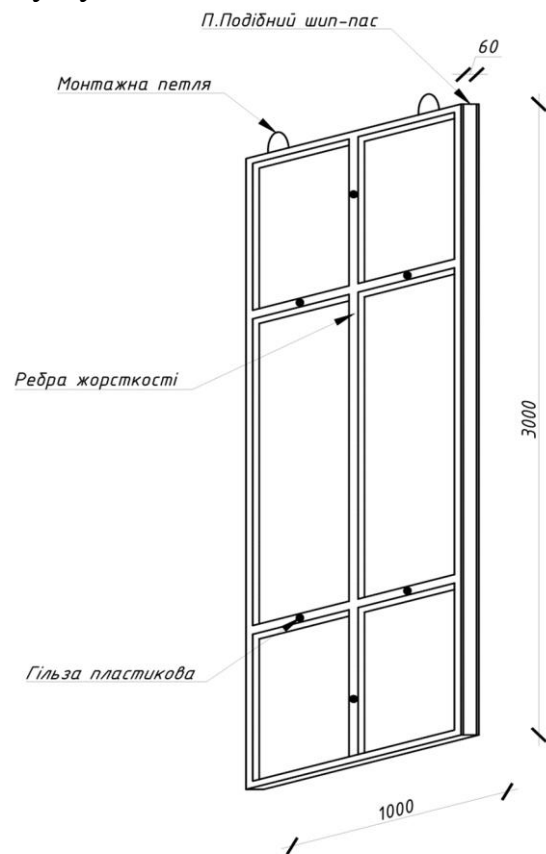
Рис. 3. Пластиковая опалубка, вигляд ззаду
