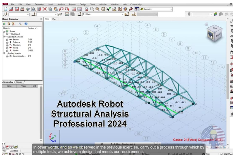
Рис. 2. Інтерфейс програми Autodesk Robot Structural Analysis Professional з моделлю порталльної рами
