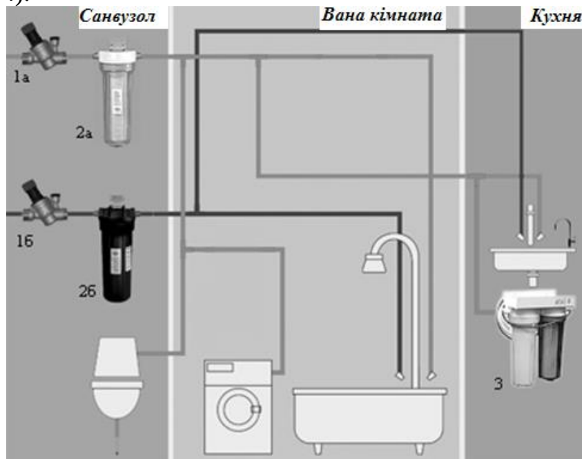
Рис. 1. Схема очищення води в квартирі (економічний варіант):
