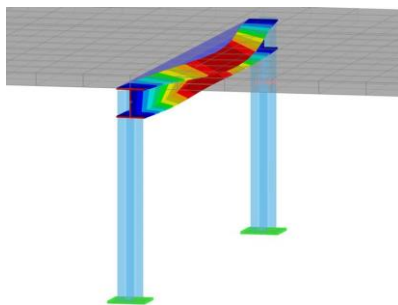
Рис. 1. Схема втрати стійкості нижнього поясу сталеві балки
