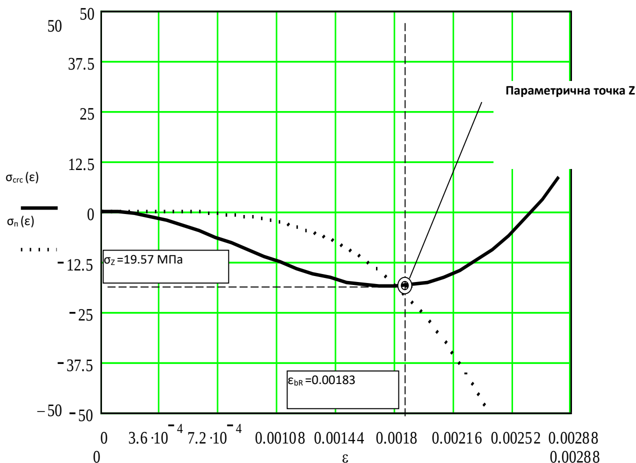
Рис. 4. Залежності \sigma_{crс}(\epsilon) і \sigma_{п}(\epsilon) , що характеризують пластичні складові напружень, та положення параметричної точки Z
