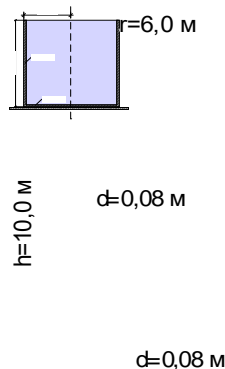
Рис. 2. Схема циліндричного резервуара з гнучким днищем на жорсткій основі.
