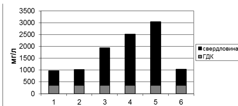
Рисуюнок 1 – Вміст хлоридів у ґрунтовій воді
