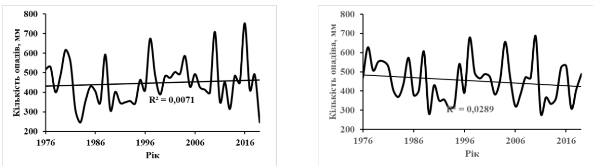
Рис.2. Динаміка річної кількості атмосферних опадів по ст. Одеса а) та ст. Херсон б) за період спостережень 1976-2019 рр.
