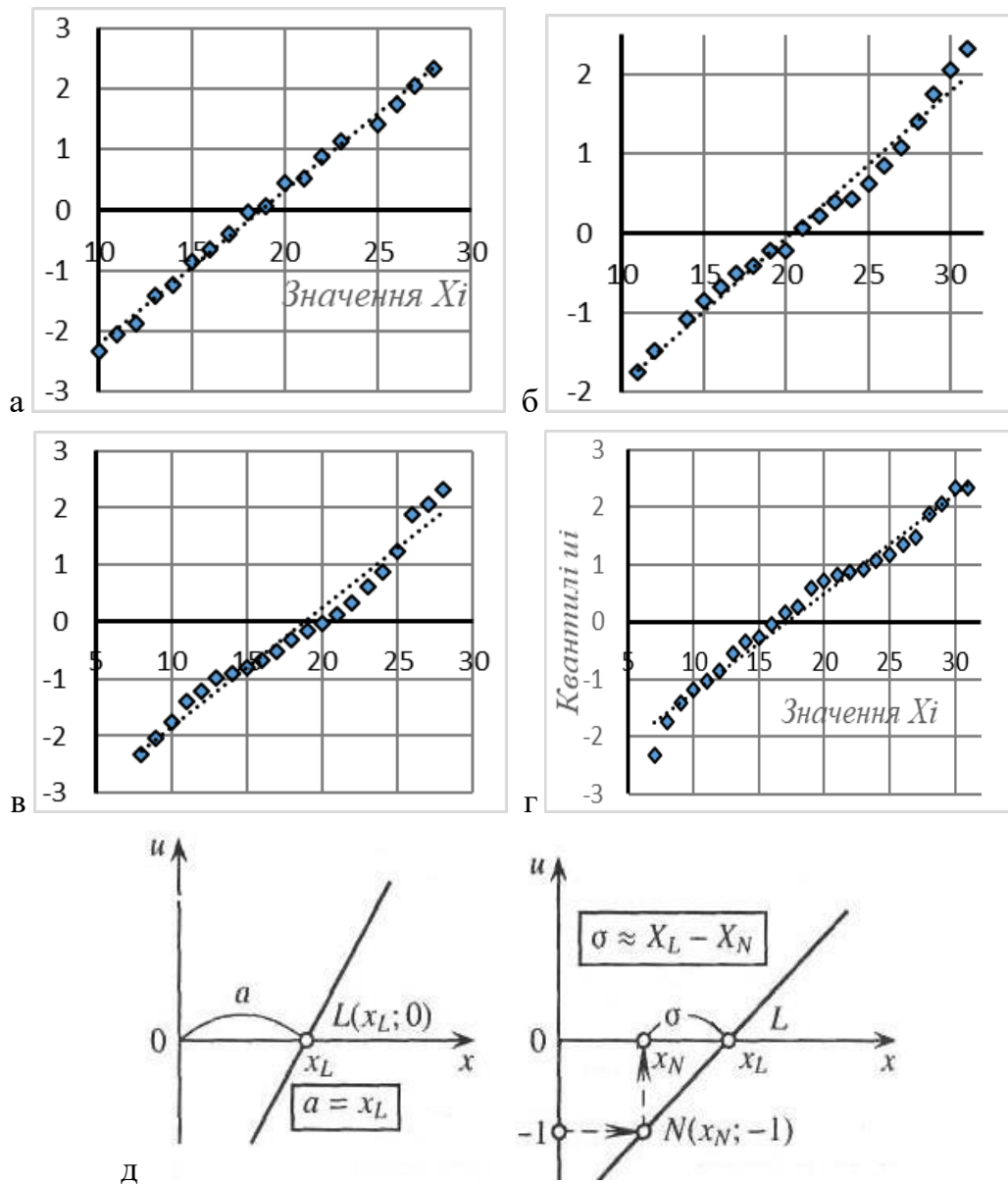
Рисунок 3. Графічна перевірка відповідності даних з радіовипромінювання нормальному закону розподілу а – схід; б – південь; в – захід; г – північ; д – розрахункова схема визначення параметрів розподілу a і \sigma [4]
