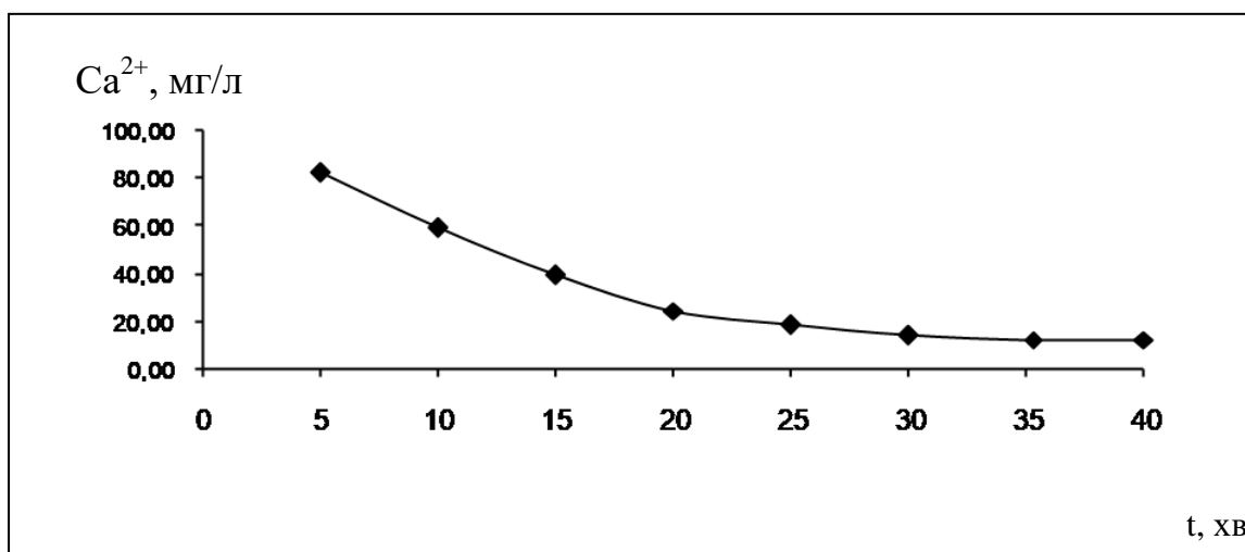
Рисунок 2. Графік сорбції розчиненого \text{Ca}^{2+} в дистильованій воді
