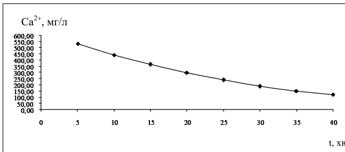
Рисунок 3. Графік сорбції \text{Ca}^{2+} у сухому стані та пропуск дистильованої води
